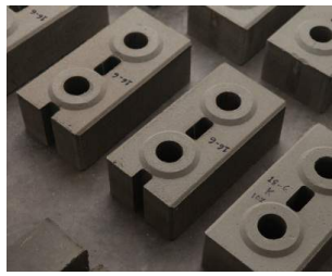
CSEB Interlocking Block
