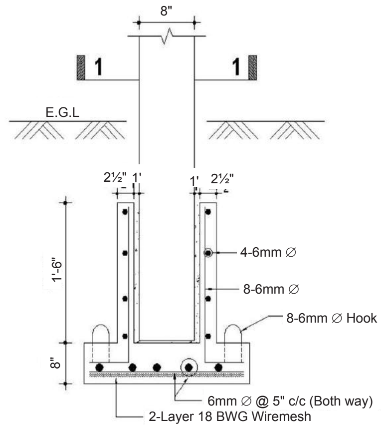
Section A-A
