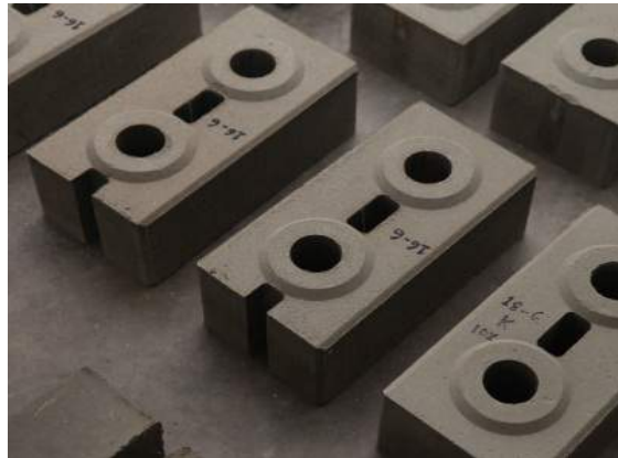
Interlocking CSEB Block
