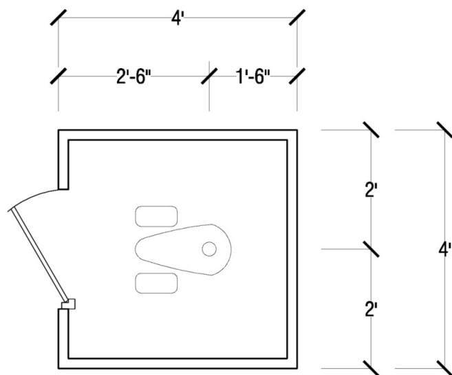
Toilet plan
