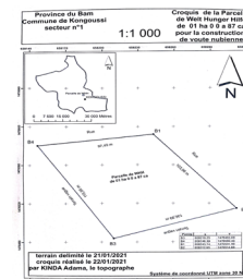
Croquis de la parcelle pour la construction de voute
