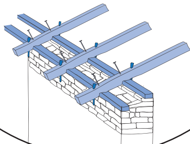
छाना र दलिनको जोडाई #१
