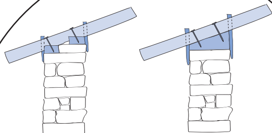
छाना र दलिनको जोडाई #१
